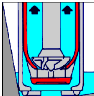
底阀开启 - 泵送液体
