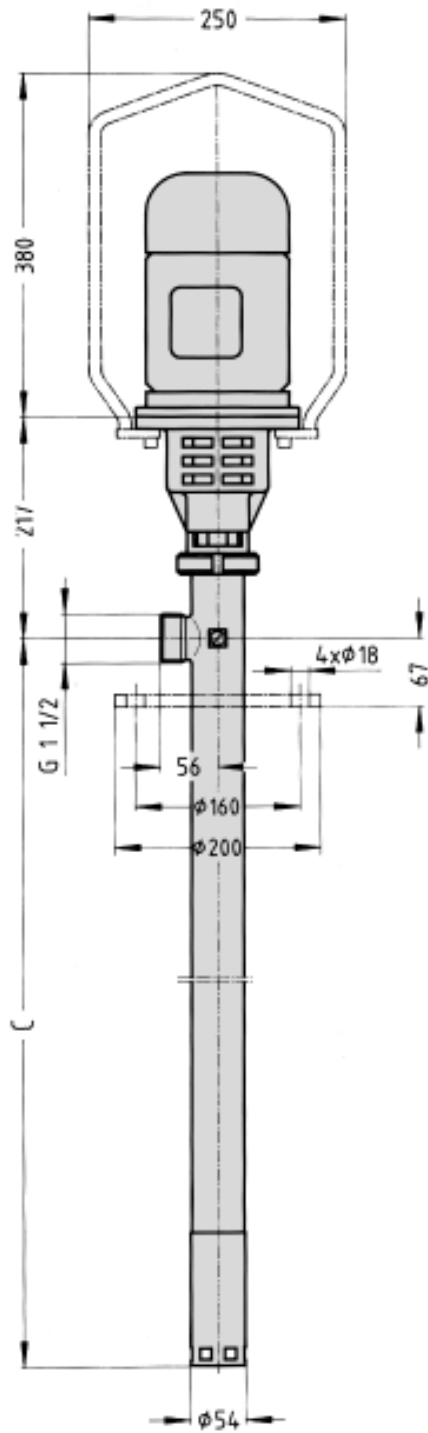
螺杆泵B70V12.1-50.1(三相马达) 尺寸图
