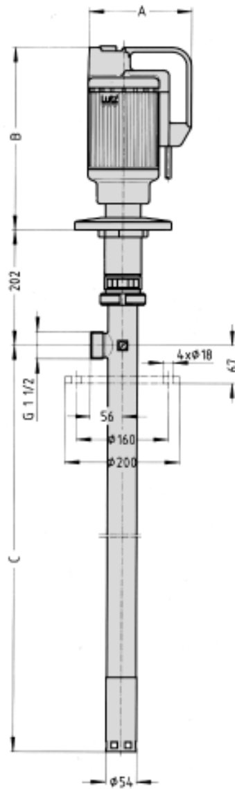
螺杆泵B70V-SR12.1-50.1 尺寸图
