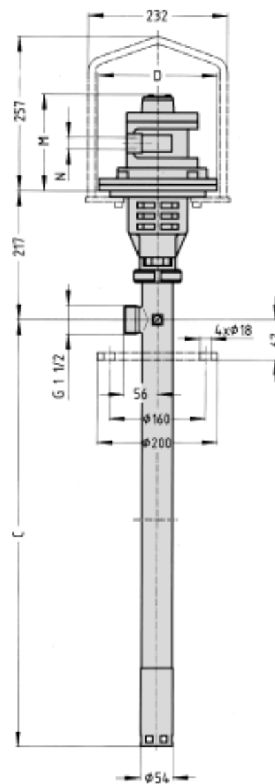
螺杆泵B70V-12.1-50.1(气动) 尺寸图
