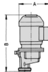
B4/GT 三相齿轮马达
