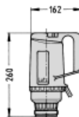
通用马达MI 4
